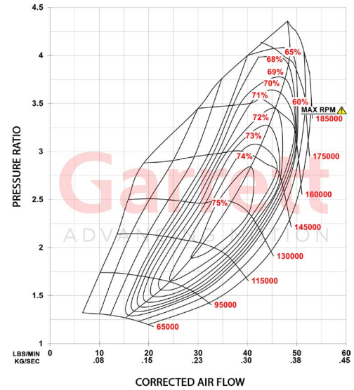
G25-585 Compressor Map
